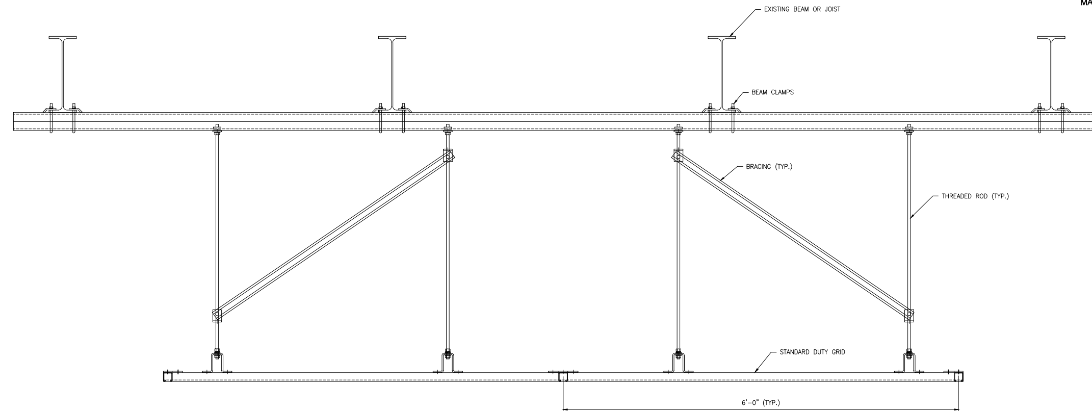
VIEW 2 SCALE: 1 1/2"=1'-0"
