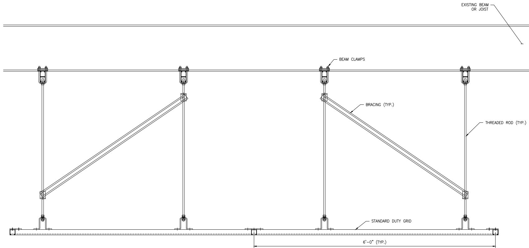
VIEW 1 SCALE: 1 1/2"=1'-0"
