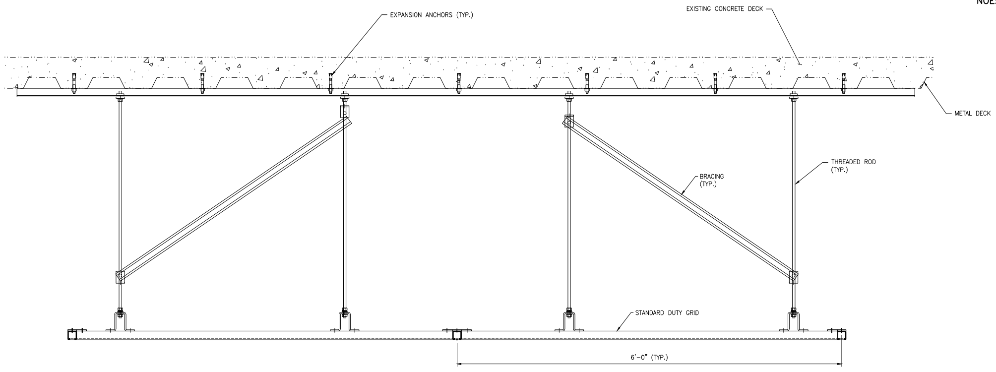
VIEW 2 SCALE: 1/2"=1'-0"
