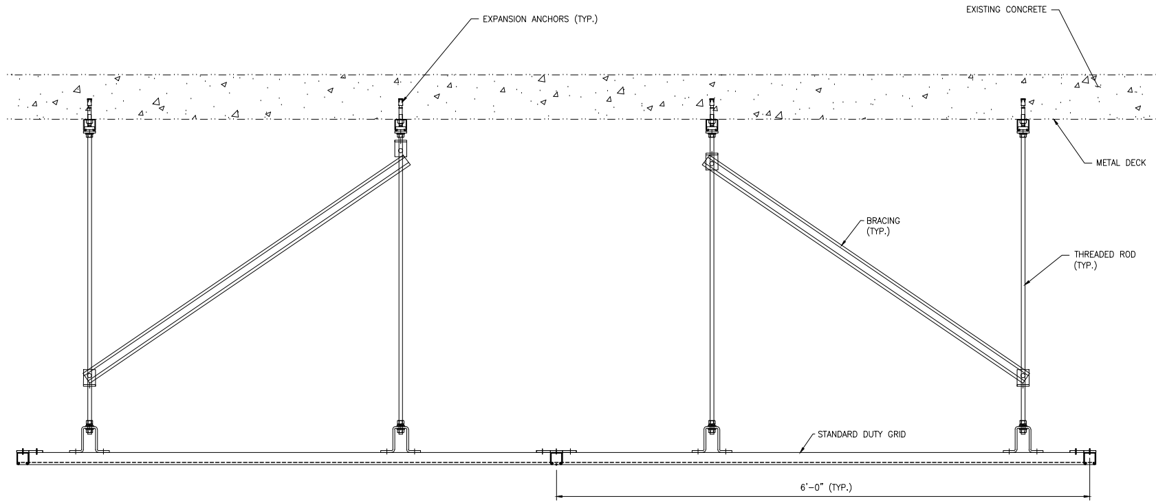
VIEW 1 SCALE: 1/2"=1'-0"
