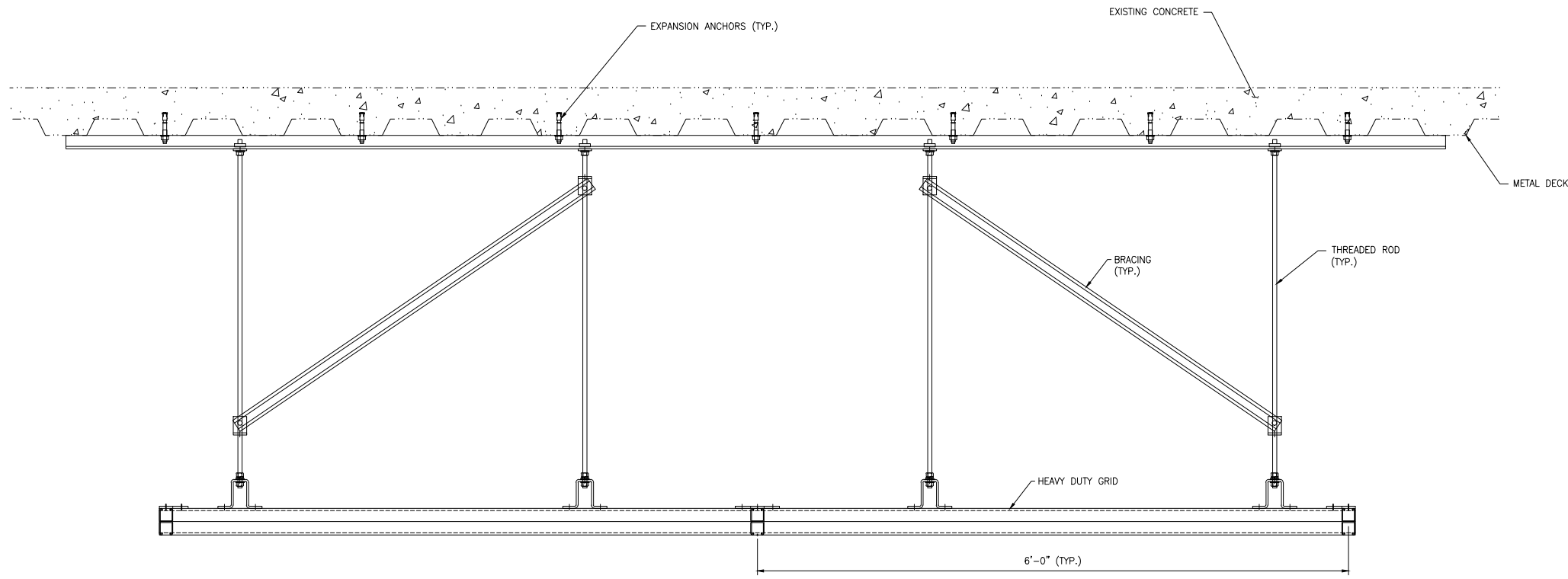
VIEW 2 SCALE: 1 1/2"=1'-0"
