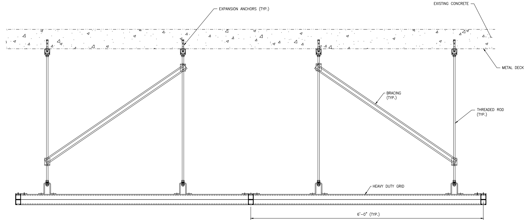
VIEW 1 SCALE: 1 1/2"=1'-0"
