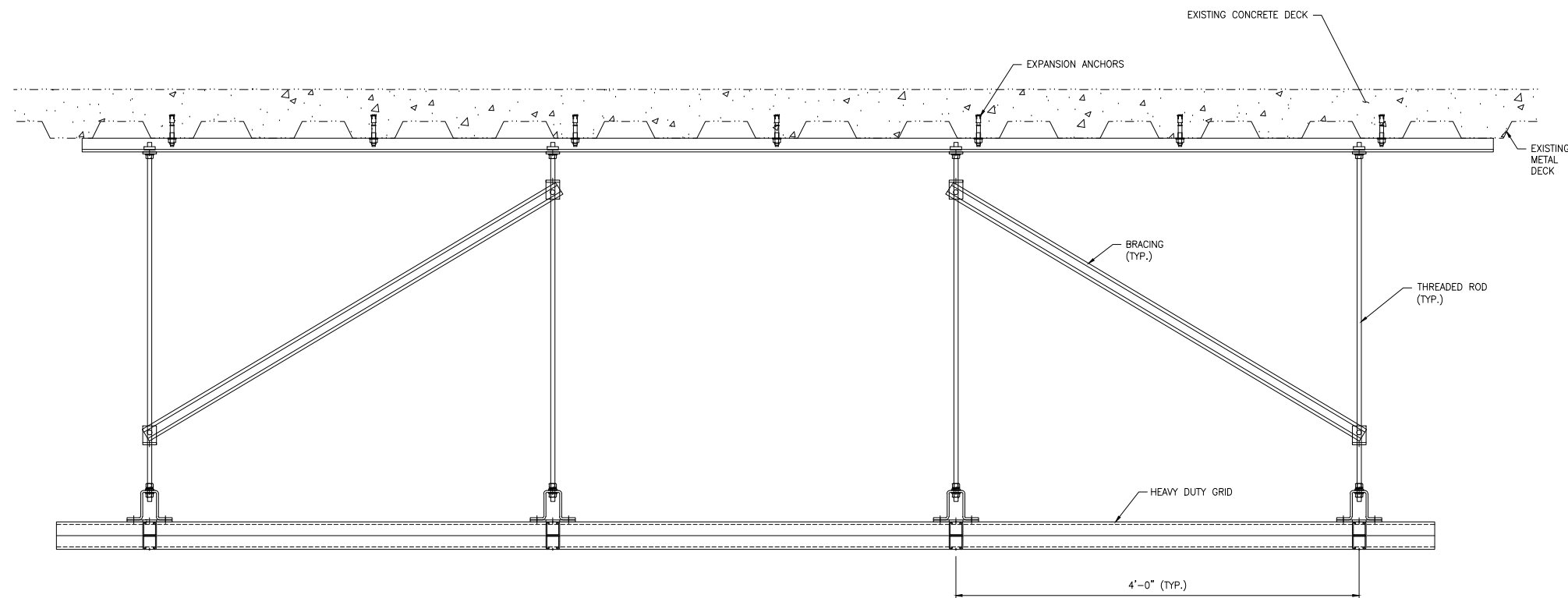
VIEW 2 SCALE: 1 1/2"=1'-0"
