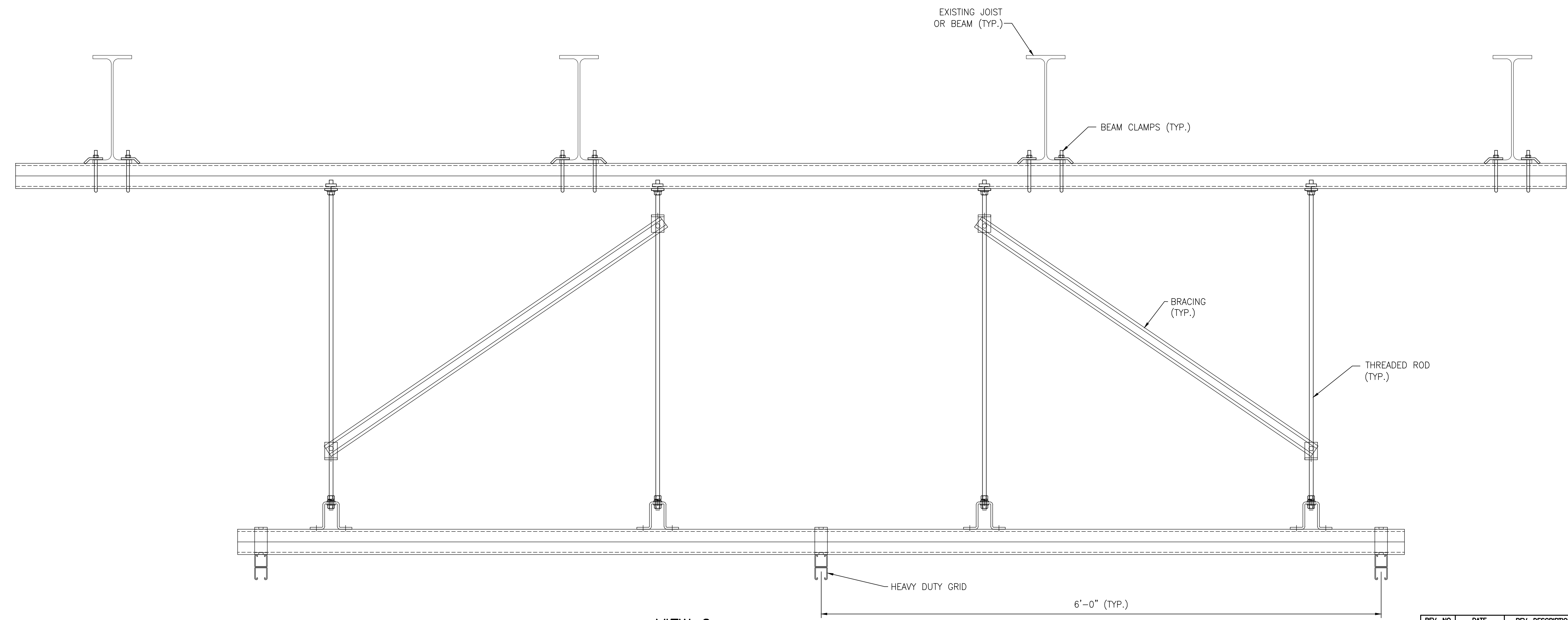
VIEW 2 SCALE: 1 1/2"=1'-0"
