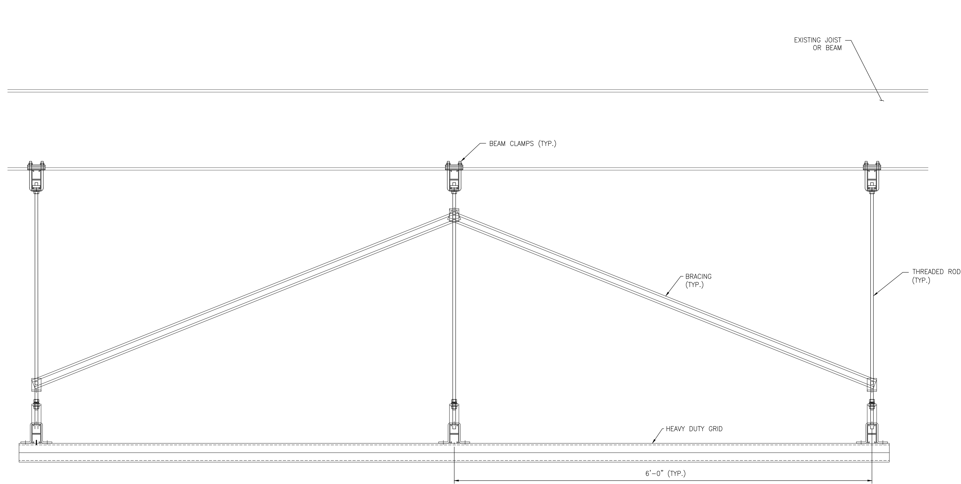
VIEW 1 SCALE: 1 1/2"=1'-0"
