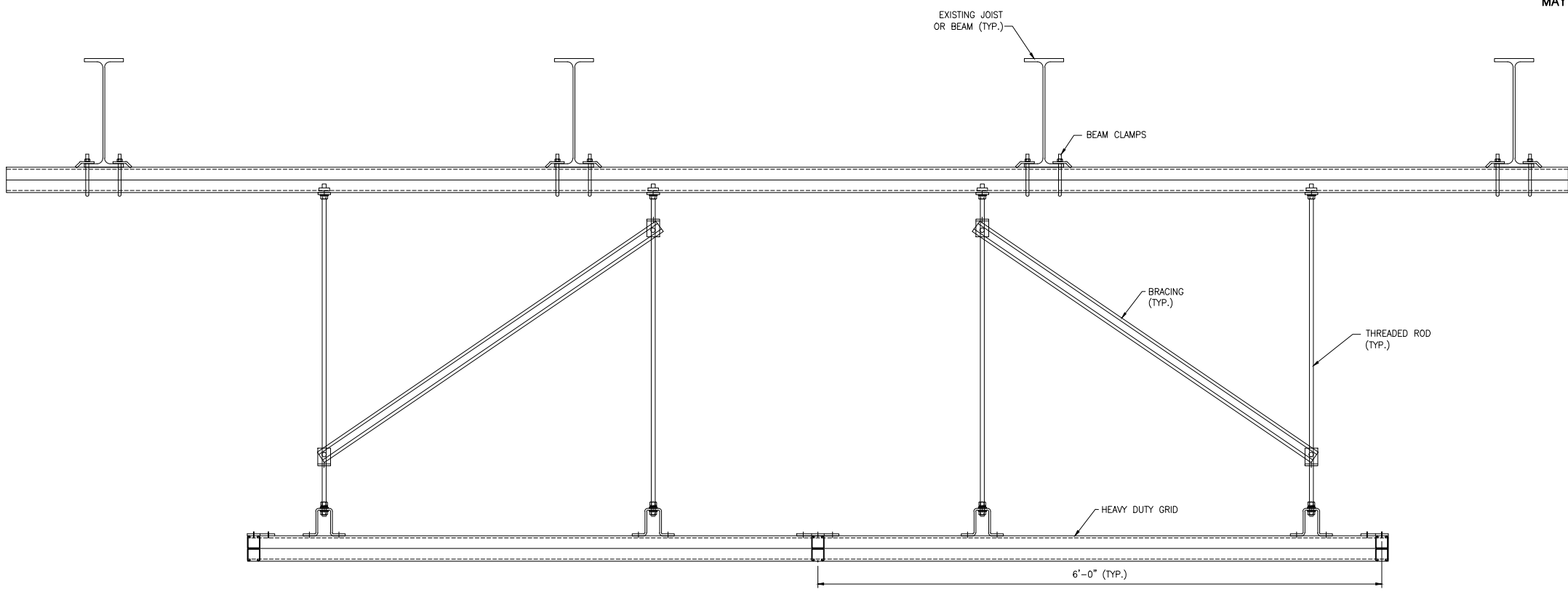
VIEW 2 SCALE: 1 1/2"=1'-0"
