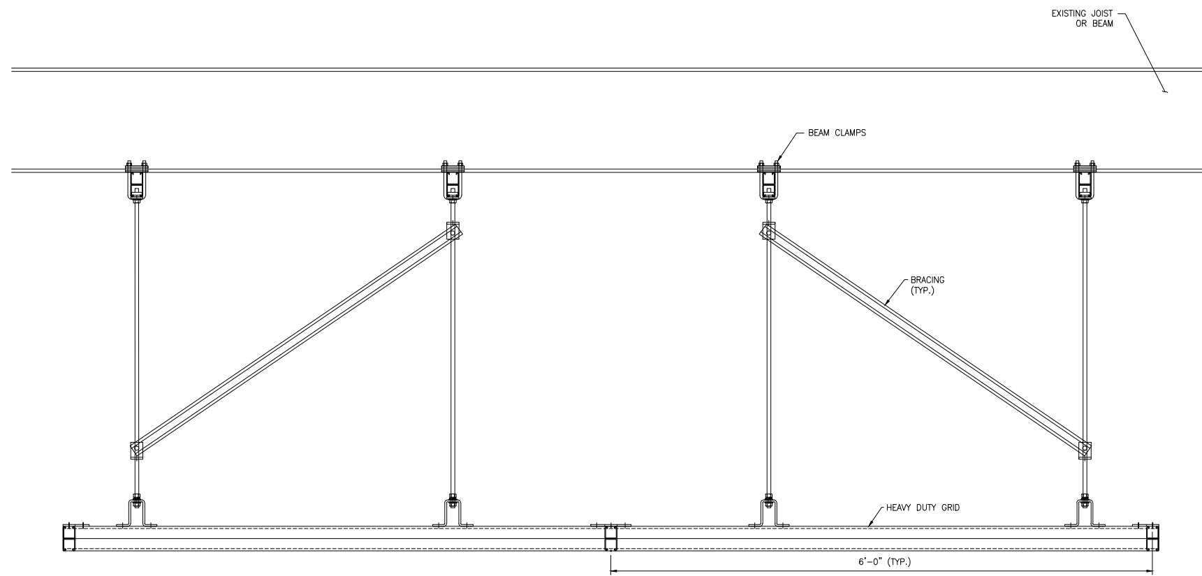
VIEW 1 SCALE: 1 1/2"=1'-0"
