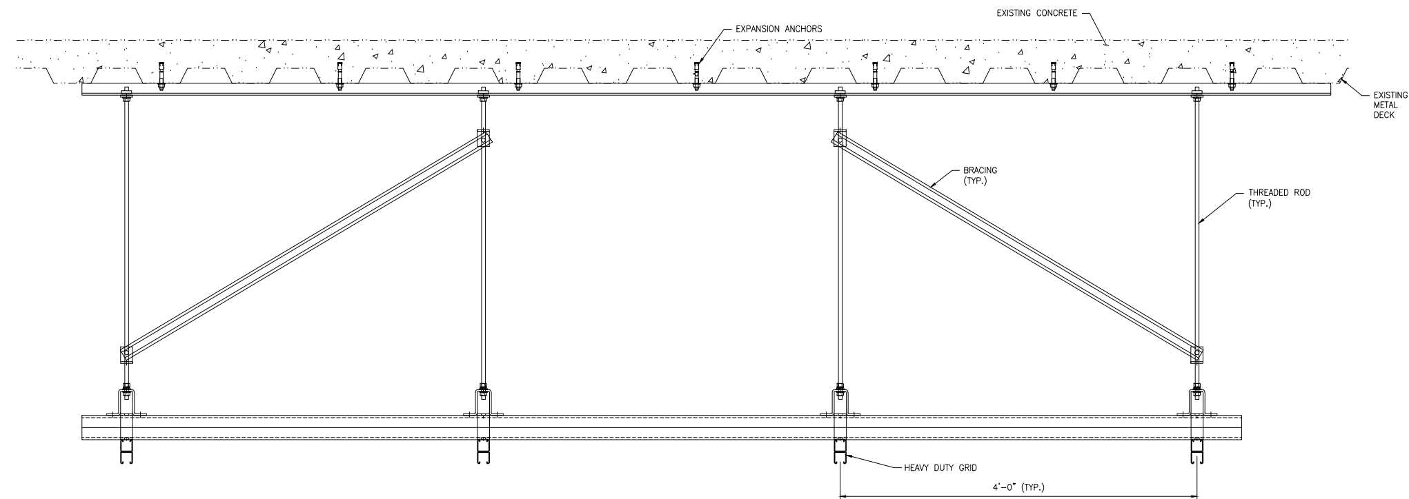
VIEW 2 SCALE: 1 1/2"=1'-0"
