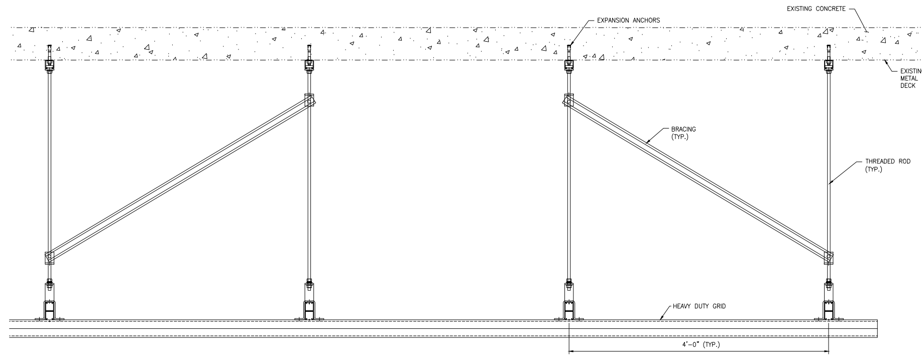
VIEW 1 SCALE: 1 1/2"=1'-0"
