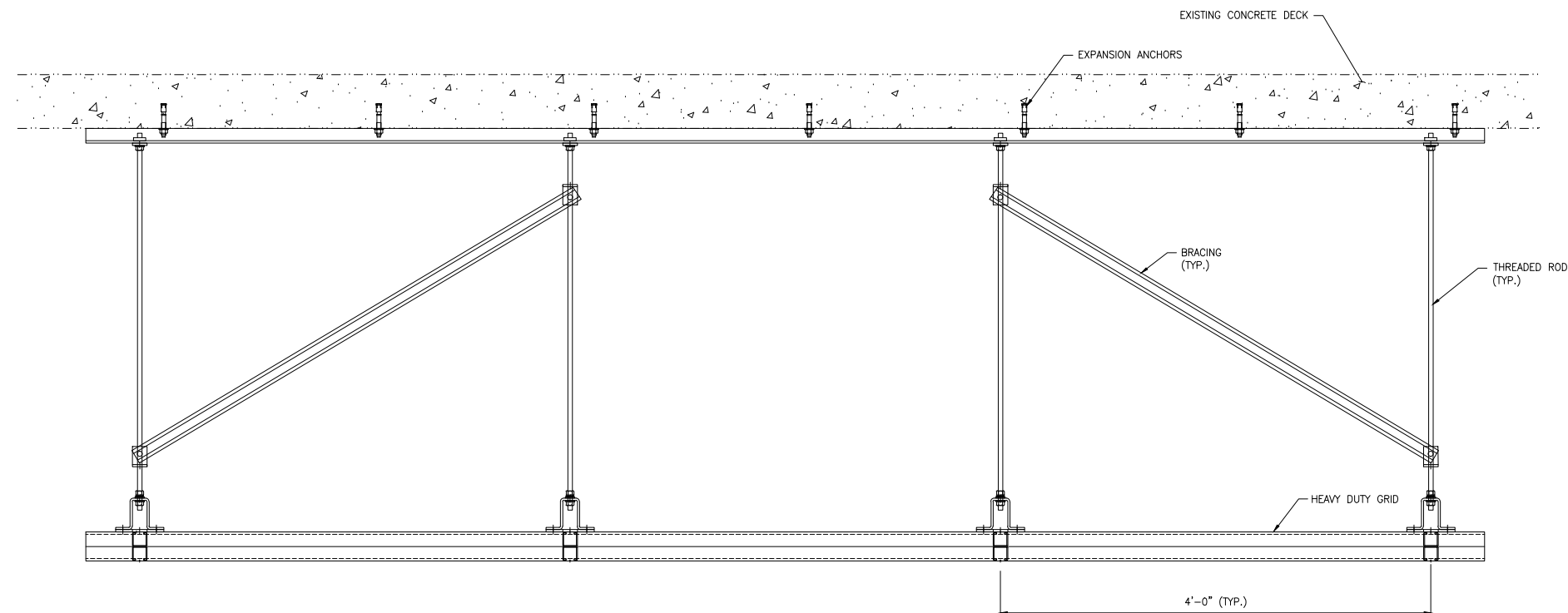
VIEW 2 SCALE: 1 1/2"=1'-0"
